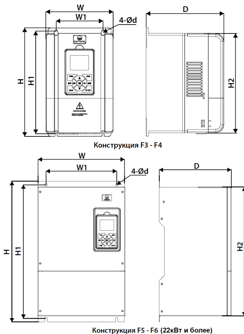
Рисунок 3.2 Габаритные размеры
