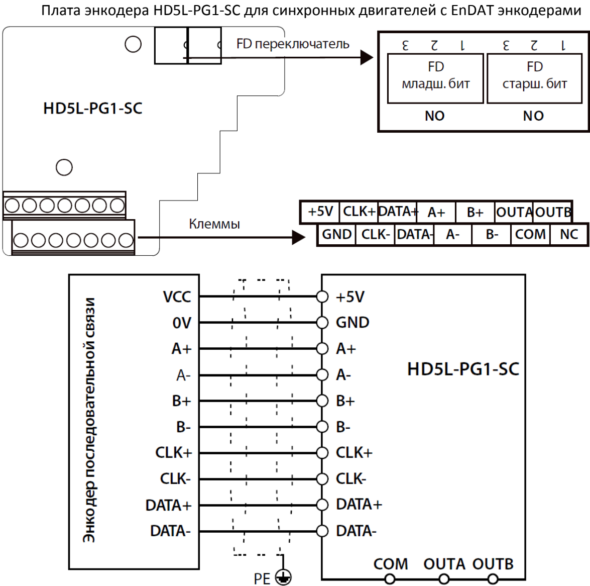
Рисунок 5.8 – Плата подключения энкодера HD5L-PG1-SC
