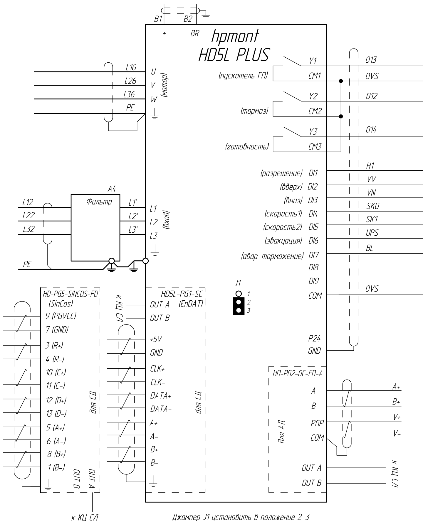
Рисунок 5.5 – Схема подключения к устройству управления СЛ
