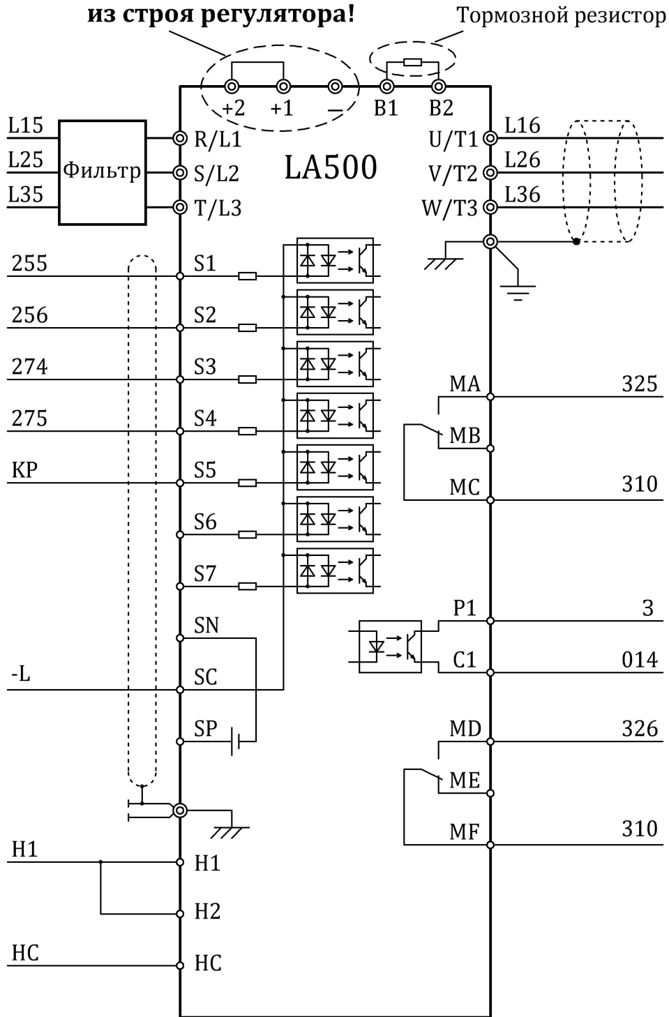
Рисунок 4.3 - Подключение к станции УЛ грузовой
